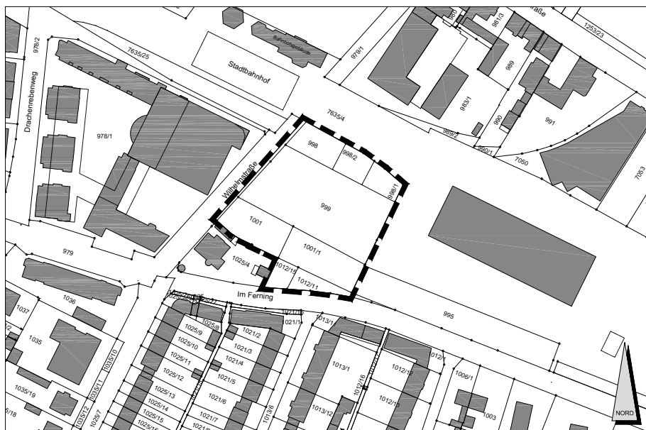
Übersichtslageplan: Vorhabenbezogener Bebauungsplan "Wilhelmstraße Ost" Planungsamt Ettlingen 21.04.2017
